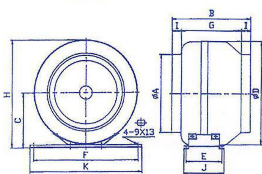
DIAMENSION(mm) 尺寸
